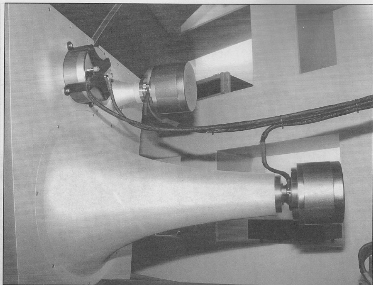
Ultimate II 的號角固然是精密級「全鋁打」，而單元亦全屬現下最頂級的鋼磁出品。
