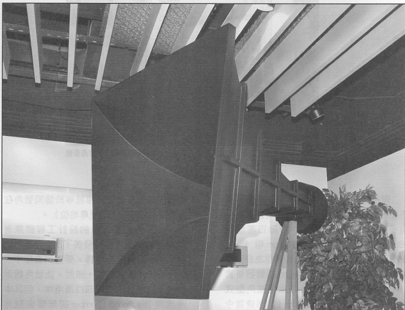
置於頂部的低音號角，以其形格計，實不下於大型古董劇院級號角。
